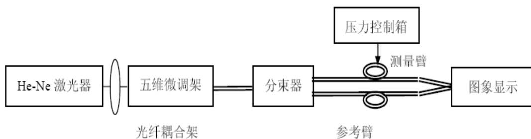
图3 压力传感原理示意图
