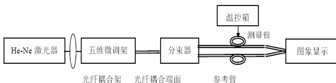
图 4 温度传感原理示意图
